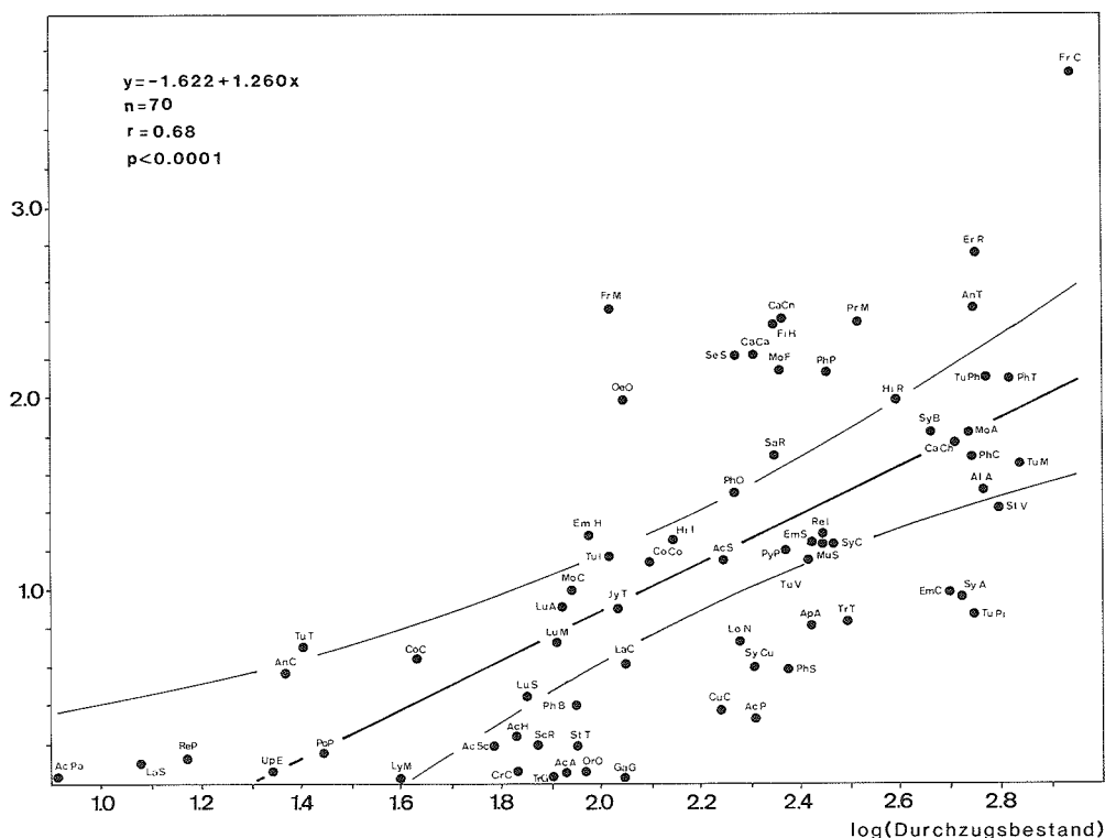
Abb.1. Beziehung zwischen dem «Durchzugsbestand», einem Mass für die erwarteten Zugvolumen über den Alpen (s. Kap.1.5. und 2.2.1.), und den mittleren jährlichen Fanghäufigkeiten von Tag- und Nacht-fänglingen auf dem Col de Bretolet. Eingetragen sind die einbezogenen 70 Arten (Abkürzungen s. Tab.3) und die Regressionsgerade mit dem 99%-Vertrauensbereich. – Relationship between a measure of expected relative numbers of migrants in Switzerland (x-axis) and the mean number of birds caught per year on Col de Bretolet during the migrating season of the species concerned. The 70 species examined, the linear regression line and the 99% confidence limits are indicated.
