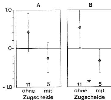
Abb.7. Mittlere Abweichungen für Arten ohne bzw. mit einer Zugscheide in Europa westlich von Russland in der Gruppe der kleinen Arten mit SW Zugrichtung in Europa, die nicht auf Feuchtgebiete angewiesen sind und nur nachts ziehen: (A) = Tag- und Nachtfänge (vgl. Abb.1). (B) = Nachtfänge (vgl. Abb.4). – Mean residuals for species without and with a migratory divide in Europe west of Russia within the group of small night migrants with a SW direction of migration in western Europe and not requiring wet habitats. (A) = day and night captures (cf. fig.1). (B) = night captures (cf. fig.4).
