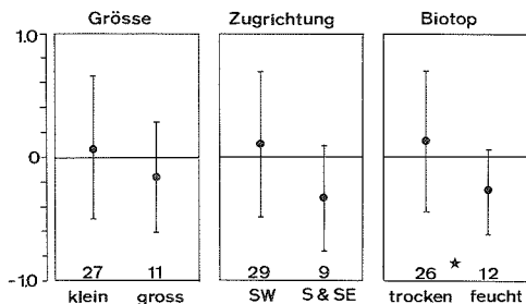
Abb.5. Mittlere Abweichungen aus der in Abb.4 dargestellten Beziehung (Nachtfänge) für verschiedene Artengruppen (wie Abb.2). – Mean residuals (from fig.4, night captures) for various groups of species (as fig.2).
