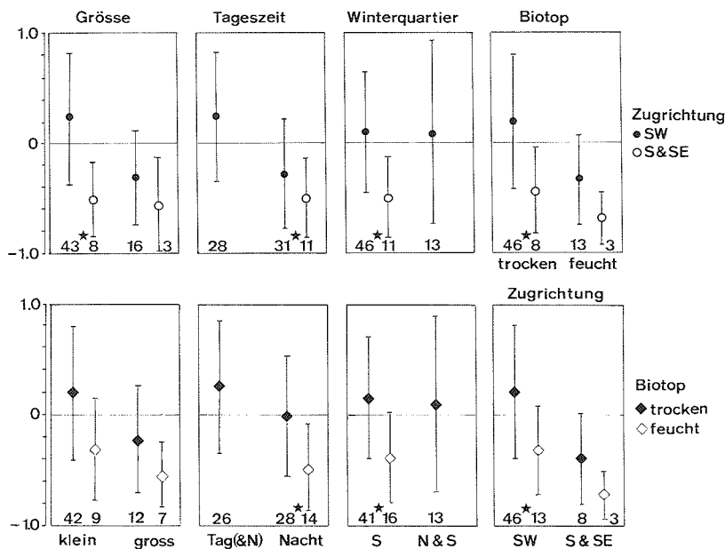
Abb. 3. Mittlere Abweichungen aus der in Abb. 1 dargestellten Beziehung für verschiedene Artengruppen, die zusätzlich nach der Zugrichtung in Europa (oben) und nach dem Biotopanspruch (unten) aufgeteilt sind (wie Abb. 2). – Mean residuals (from fig. 1) for various groups of species further split up after their direction of migration (upper row) and their habitat (lower row); see fig. 2.
