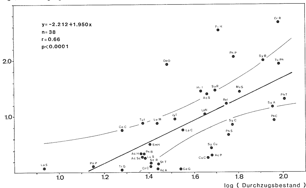
Abb.4. Beziehung zwischen dem «Durchzugsbestand der Nachtzieher» und den mittleren jährlichen Nachtfanghäufigkeiten auf Col de Bretolet für ausschliesslich nachts ziehende Arten (wie Abb.1). – Relationship between the measure of expected relative numbers of night migrants in Switzerland (x-axis) and the mean annual number of birds caught on Col de Bretolet during night (as fig.1).
