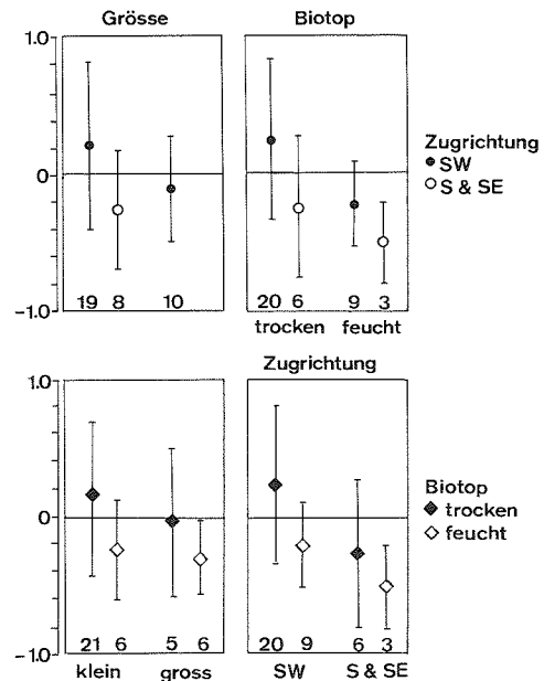
Abb.6. Mittlere Abweichungen aus der in Abb.4 dargestellten Beziehung (Nachtfänge) für verschiedene Artengruppen, die zusätzlich nach der Zugrichtung in Europa (oben) und nach dem Biotopanspruch (unten) aufgeteilt sind (wie Abb.3). – Mean residuals (from fig.4) for various groups of species split up after their direction of migration (upper row) and their habitat (lower row); see fig.3.
